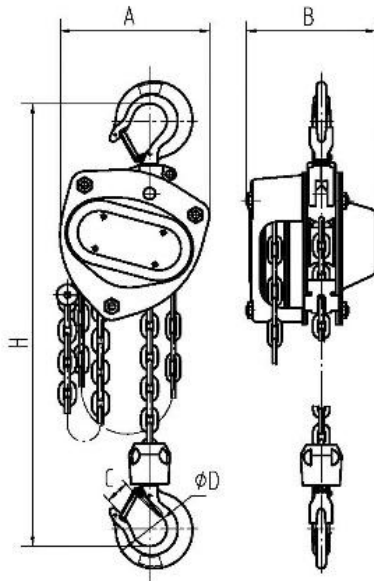
500kg – 2t
